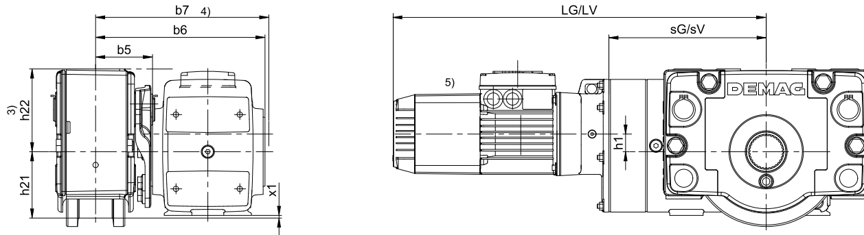
Getriebebauform: Fuß unten
