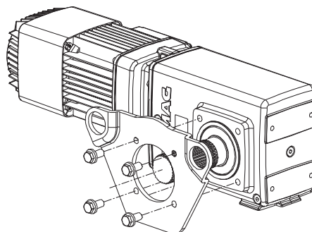
Winkelgetriebe WUE 40 – 80
