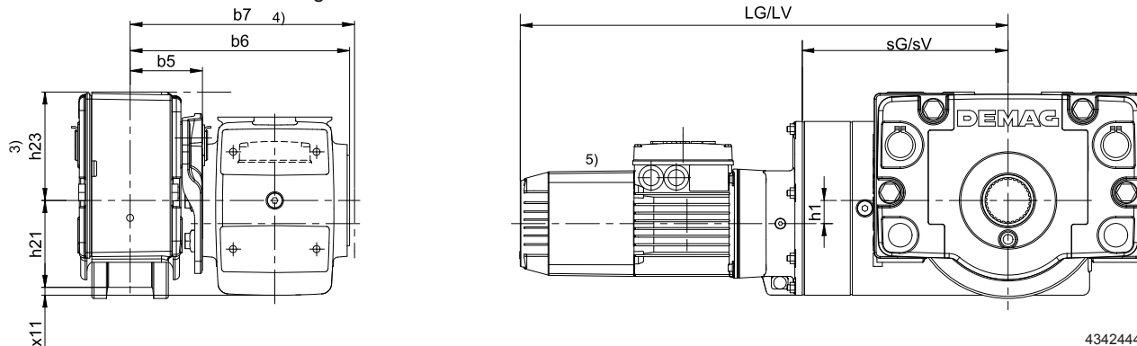
Getriebebauform: Fuß oben
