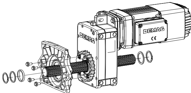
Flachgetriebe AMK 10 – 40
