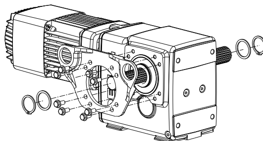
Winkelgetriebe WUK 40 – 100
