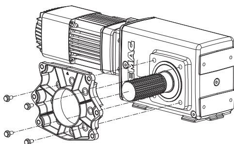
Winkelgetriebe WUK 10 – 50
