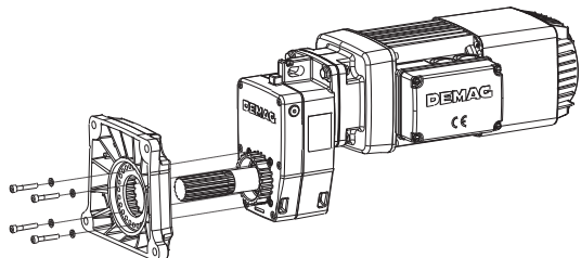
Flachgetriebe AMK 10 – 40
