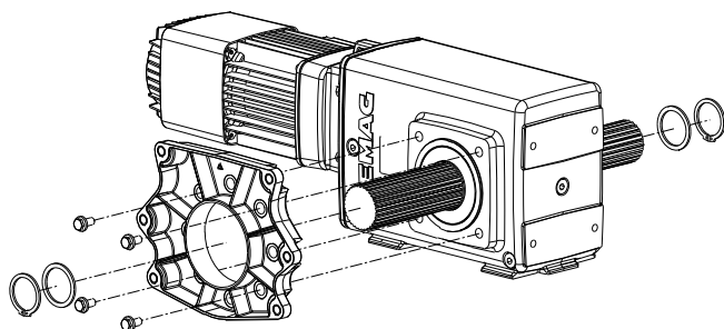
Winkelgetriebe WUK 10 – 50
